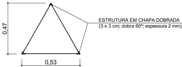
PLANTA esc.: 1:20
