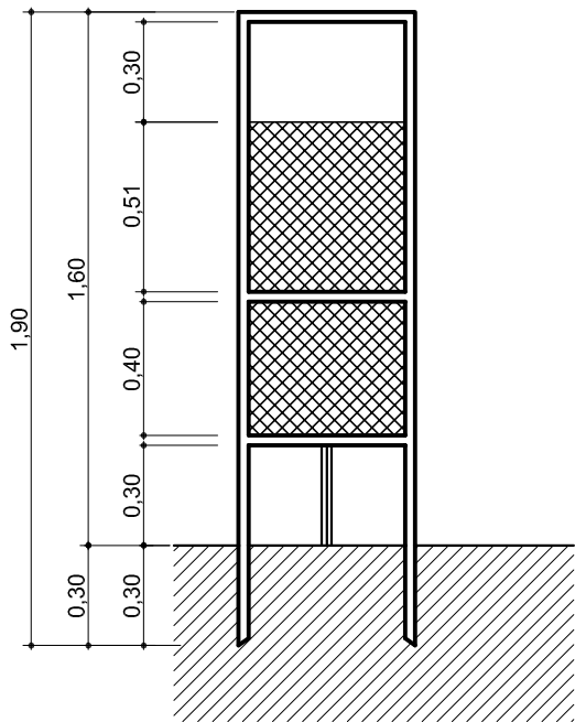
CORTE esc.: 1:25
